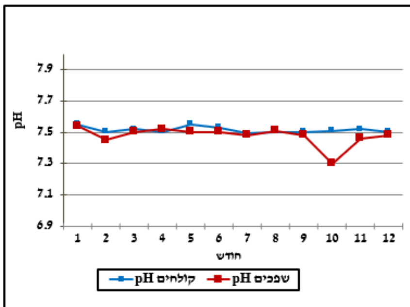
איור 14: pH בשפכים ובקולחים 2024
