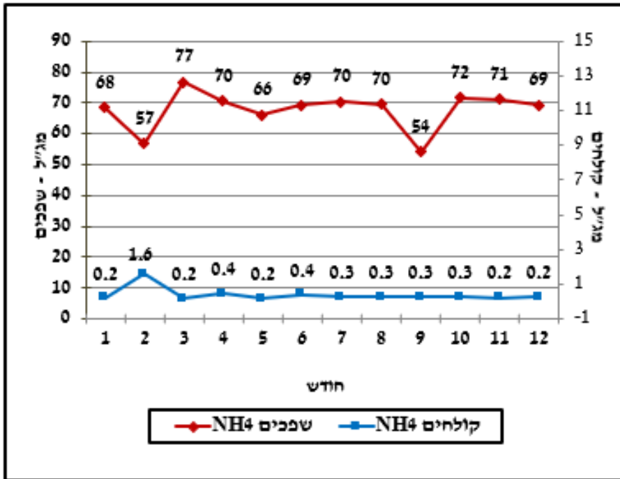
איור 12: ריכוז חנקן אמוניקלי בשפכים ובקולחים 2024
