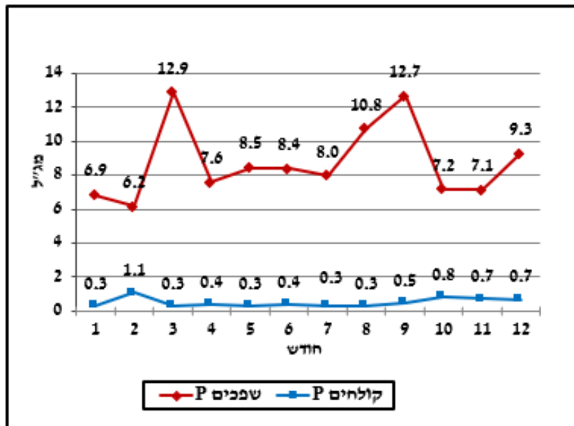
איור 11: ריכוזי זרחן (Pt) בשפכים הגולמיים ובקולחים 2024
