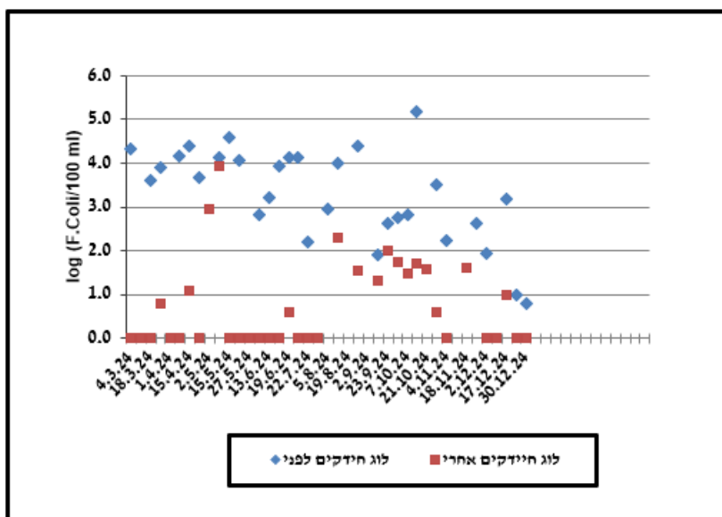
איור 16: ספירות חיידקי ק. צואתי בכניסה וביציאה מתעלת ה-UV (בלוג cfu/100ml)
