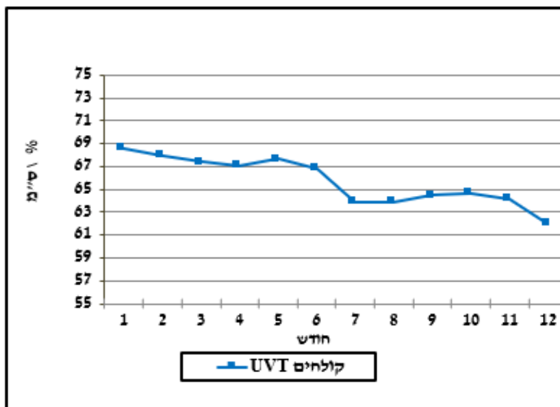
איור 15: ערכי UVI בקולחים 2024
