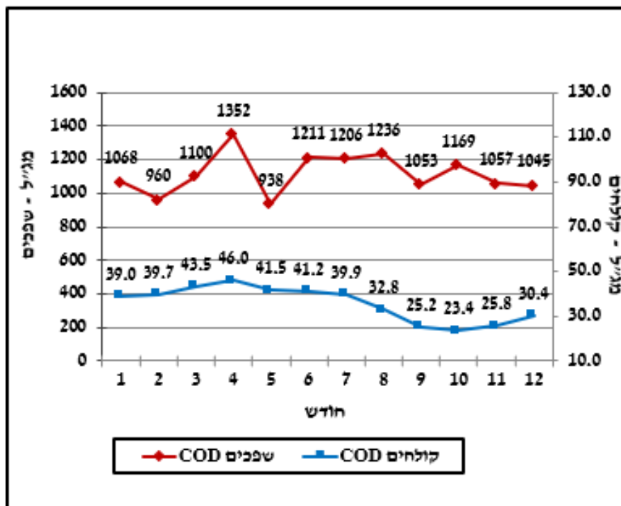
איור 9: ריכוזי צח"כ (COD) בשפכים ובקולחים 2024
