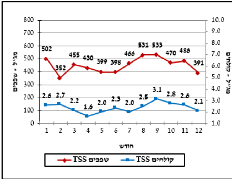
איור 10: ריכוז מוצקים מרחפים (TSS105) בשפכים ובקולחים 2024
