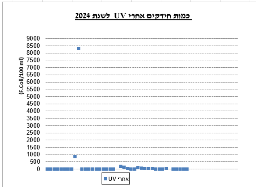
איור 17: כמות חיידקי ק. צואתי בקולחים לאחר חיטוי (cfu/100ml)
