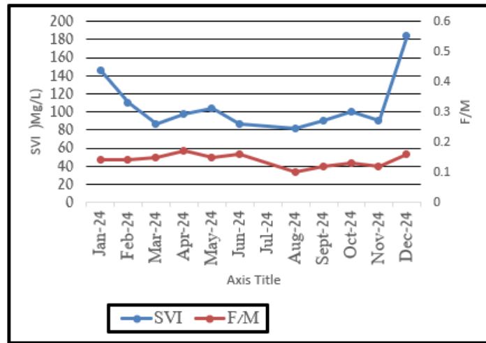
איור 6: מדד נפחיות הבוצה ויחס מזון/מיקרואורגניזמים
