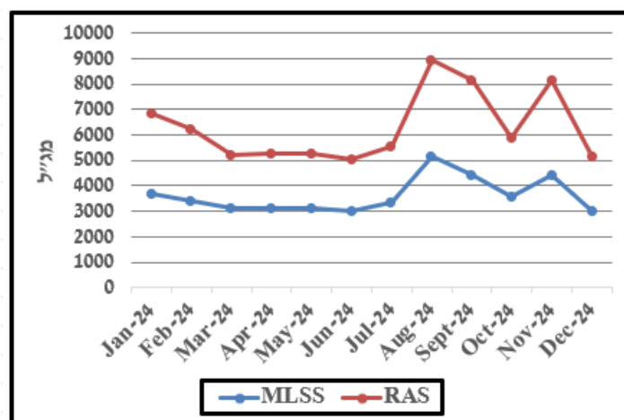
איור 5: ריכוזי נוזל מעורב ובוצה חוזרת באגני האיור מט"ש כפר סבא הוד השרון
